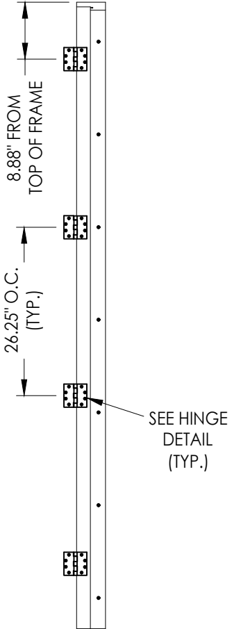
HINGE JAMB
